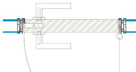
HT 1000 Holztüre 1-flügelig D = 54 mm Rw = 34 dB
