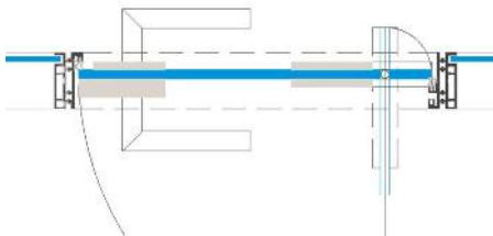
ZABA 1000 Zapfenbandtüre ESG 10 mm
