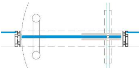
GPT 1000 Glaspandeltüre ESG 10 mm
