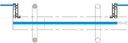
SCHAT 1000 Glasschiebetüre ESG 10 mm
