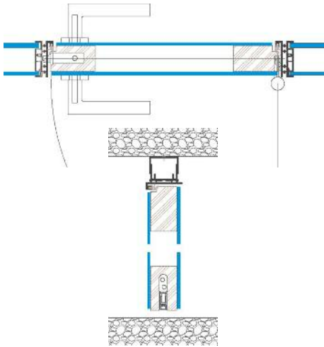
DGT 1000 Doppelglastüre 1-flügelig 2 x ESG 4 mm Rw = 36 dB
