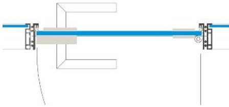
GGT 1000 Ganzglastüre ESG 10 mm Rw = 27 dB
