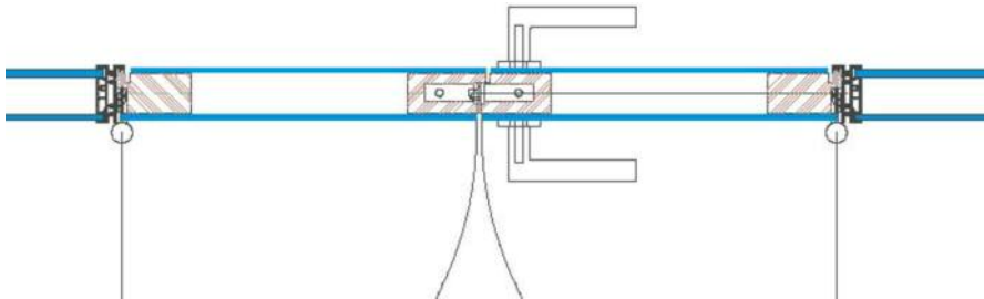
DGT2 1000 Doppelglastüre 2-flügelig 2 x ESG 4 mm Rw = 36 dB
